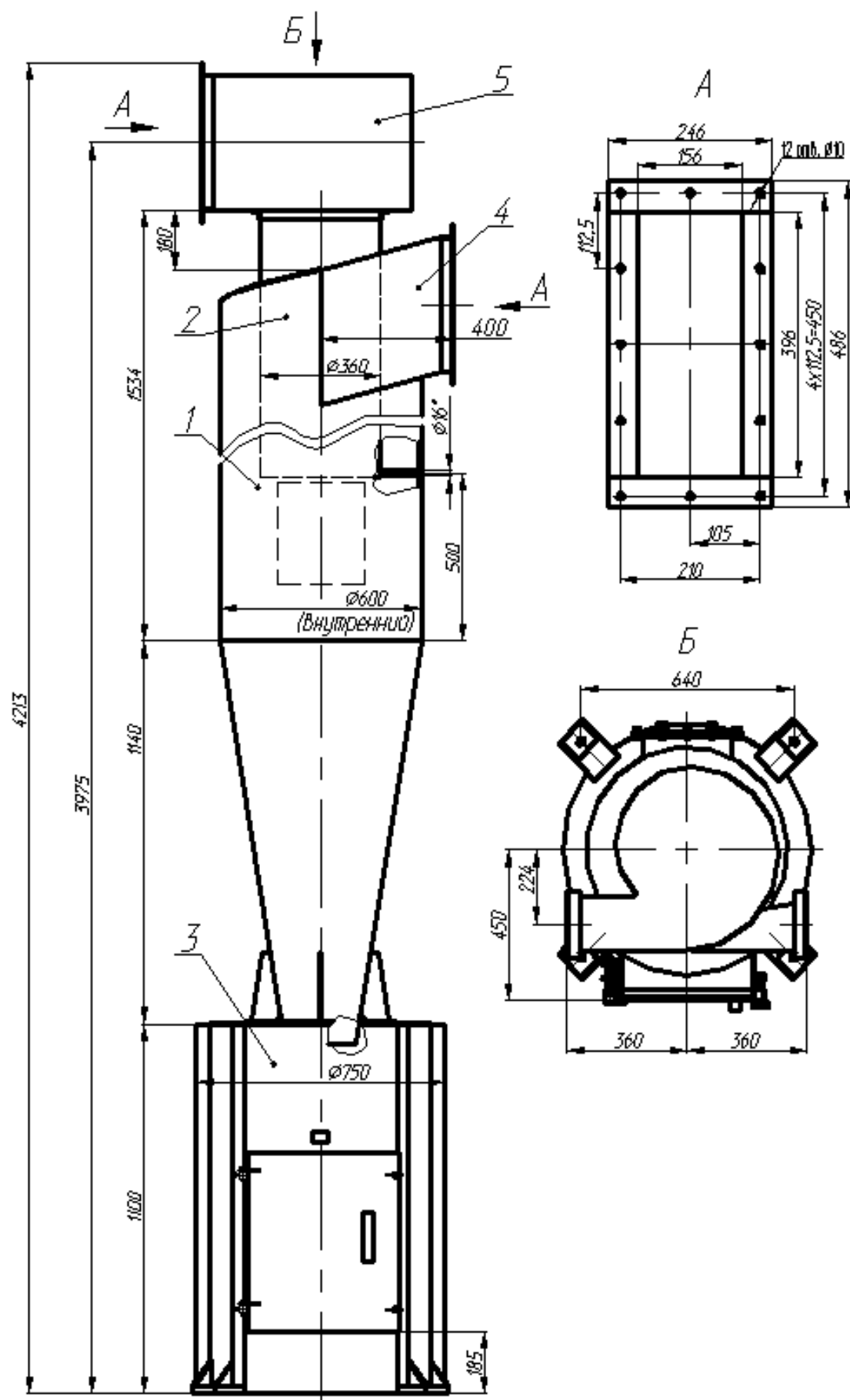
Рис.1 – Общий вид циклона ЦН 15-600 и его размеры.
