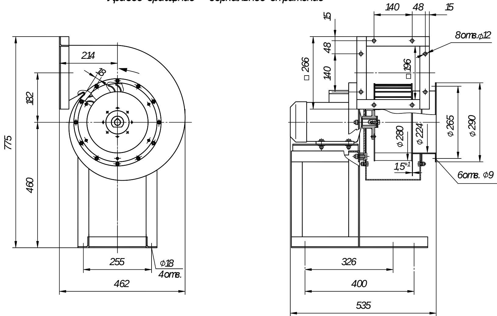
Рисунок 1 - Дымосос Д-2,8
