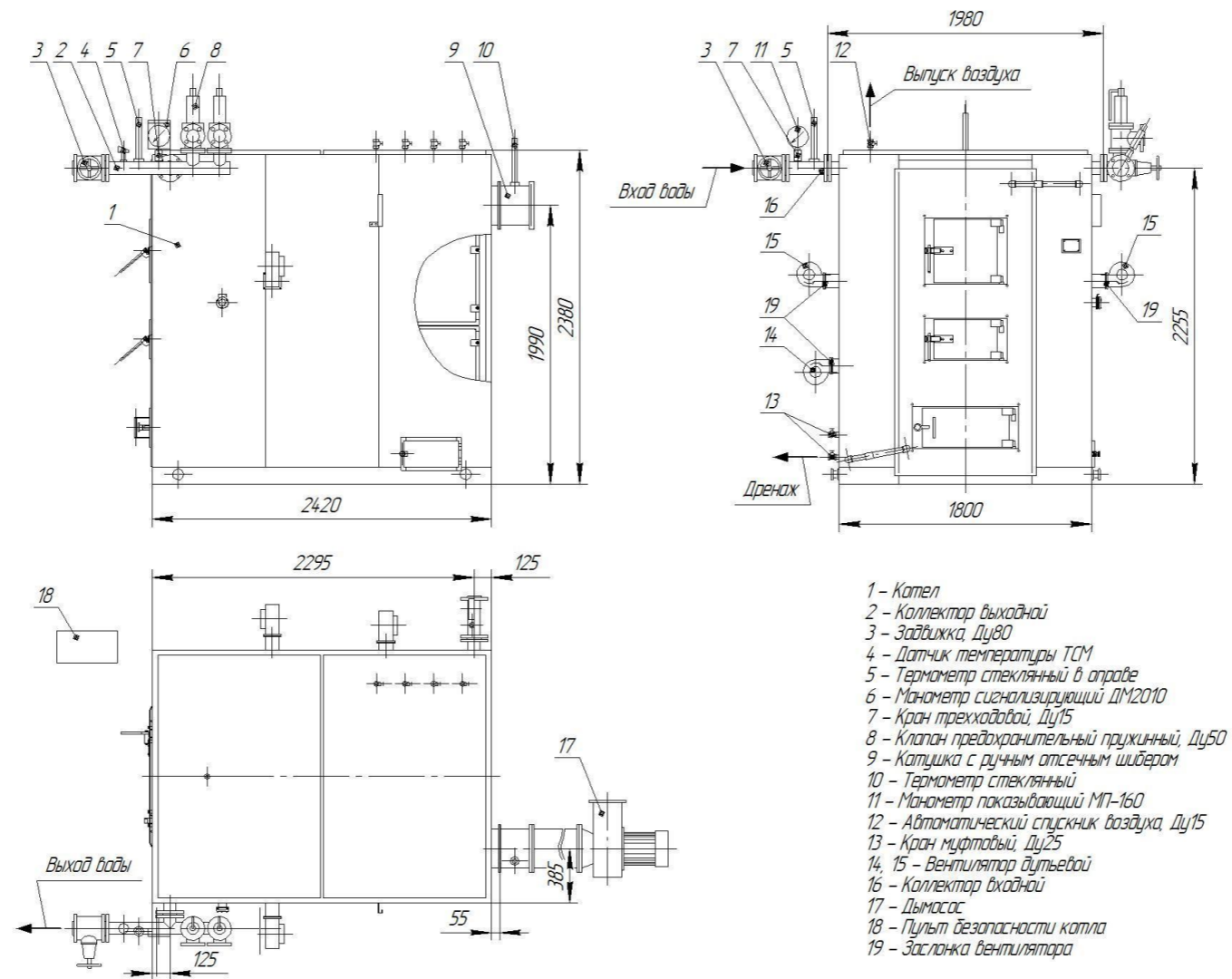
Рисунок 1 - Котел водогрейный пиролизный KB-П-0,45-95 с размещением оборудования
